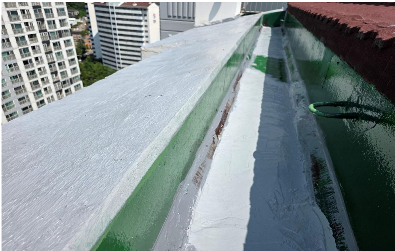
공사 중 (우레탄 중도 도포 : 배수로)
