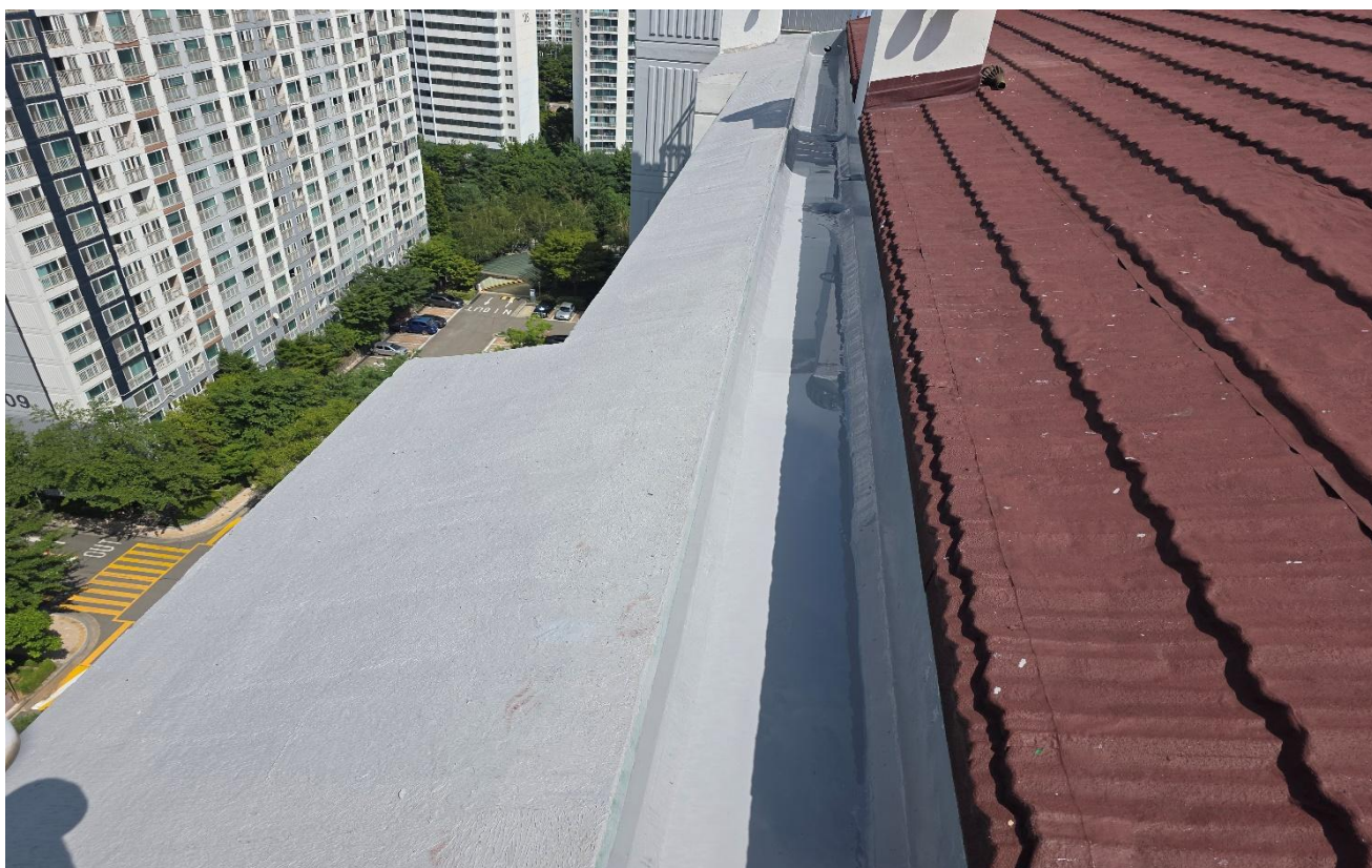
공사 중 (우레탄 중도 2차 도포 : 배수로)
