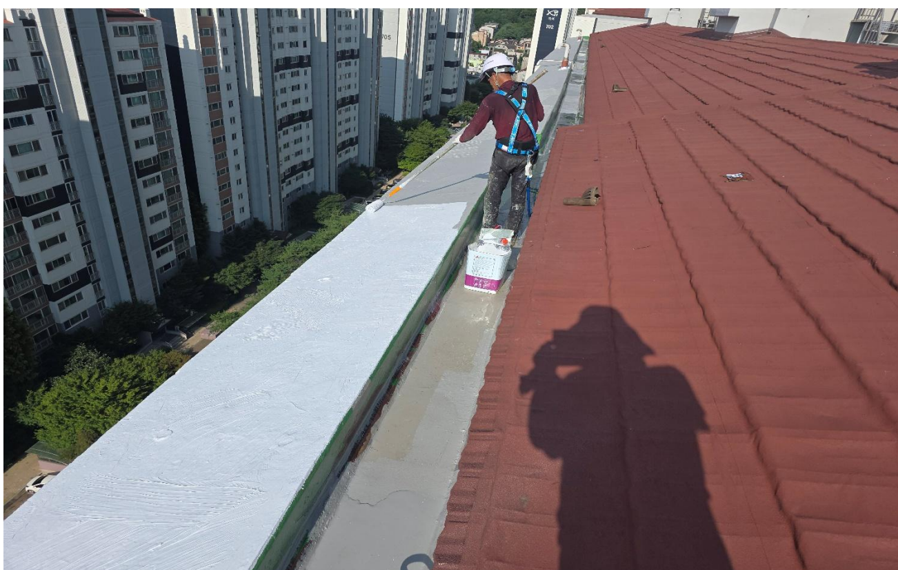
공사 중 (차열 우레탄 상도 도포 : 처마)
