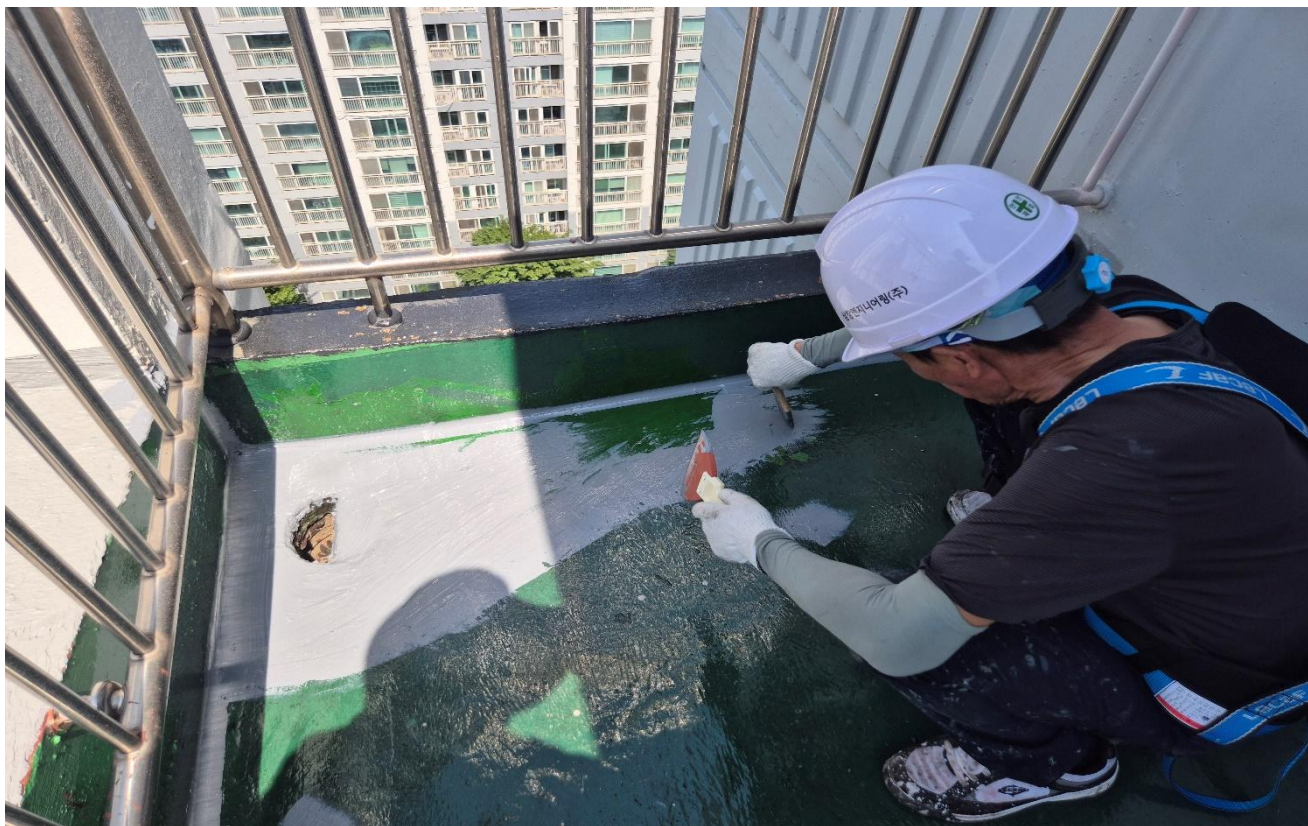
공사 중 (우레탄 실란트)
