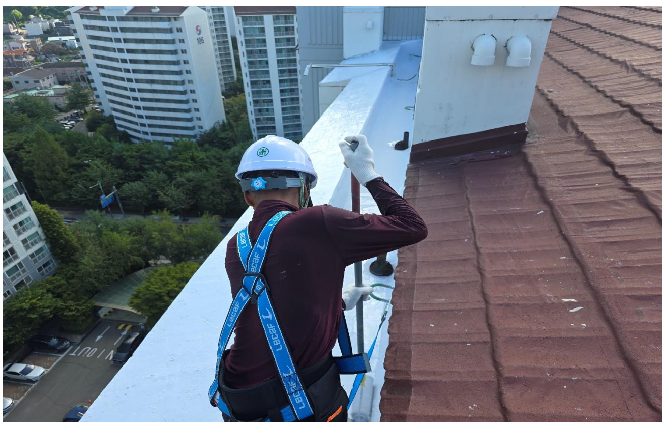
공사 중 (차열 우레탄 상도 도포 : 배수로)
