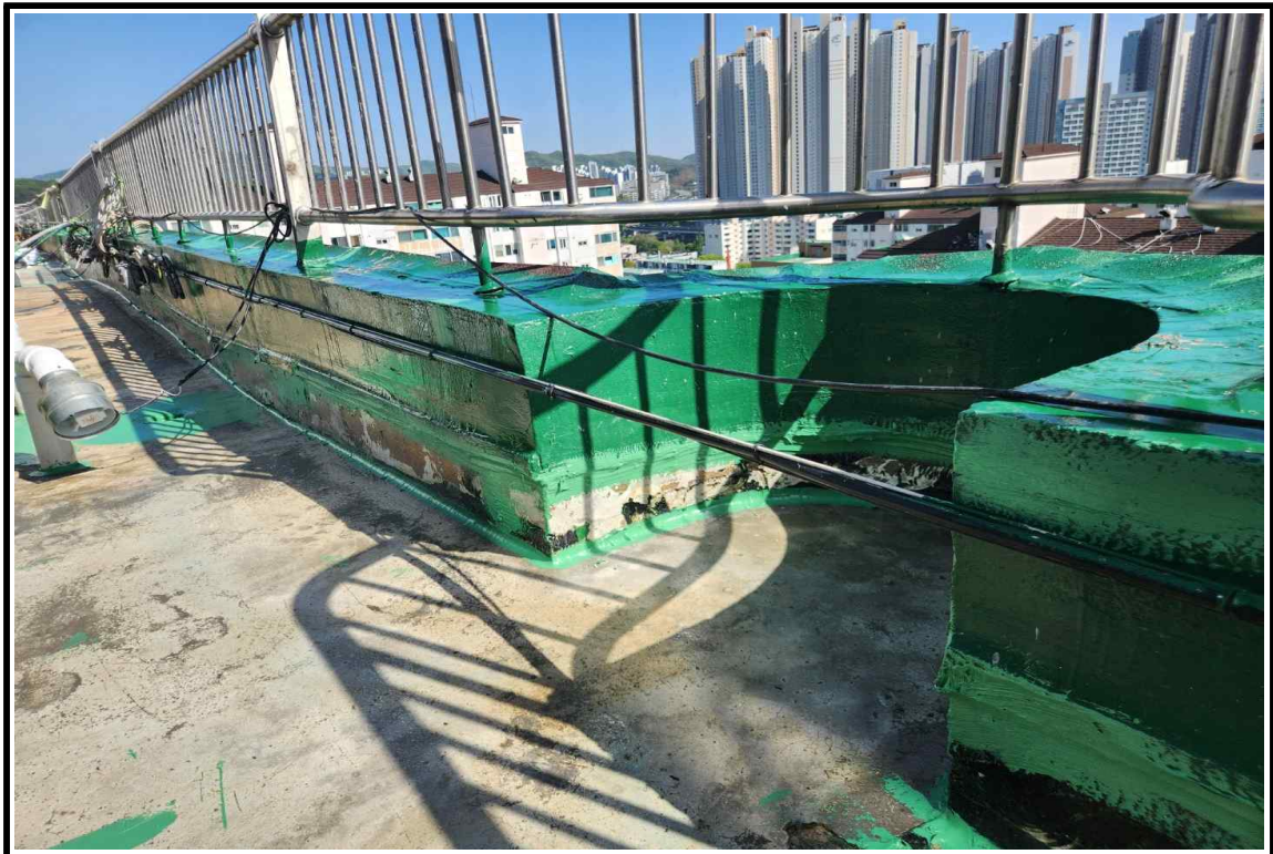
◎ 공사 중(방수공사)
