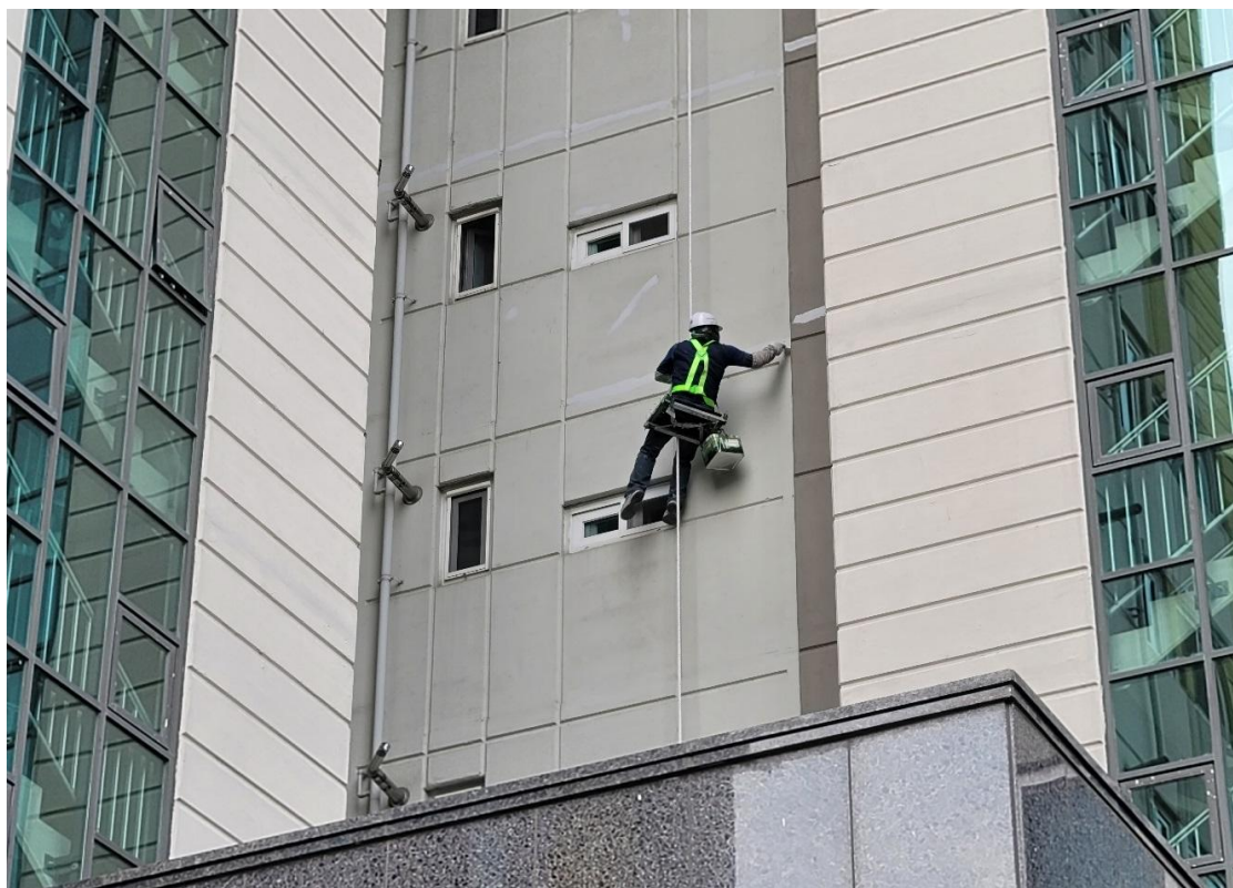
외부균열보수 1회
