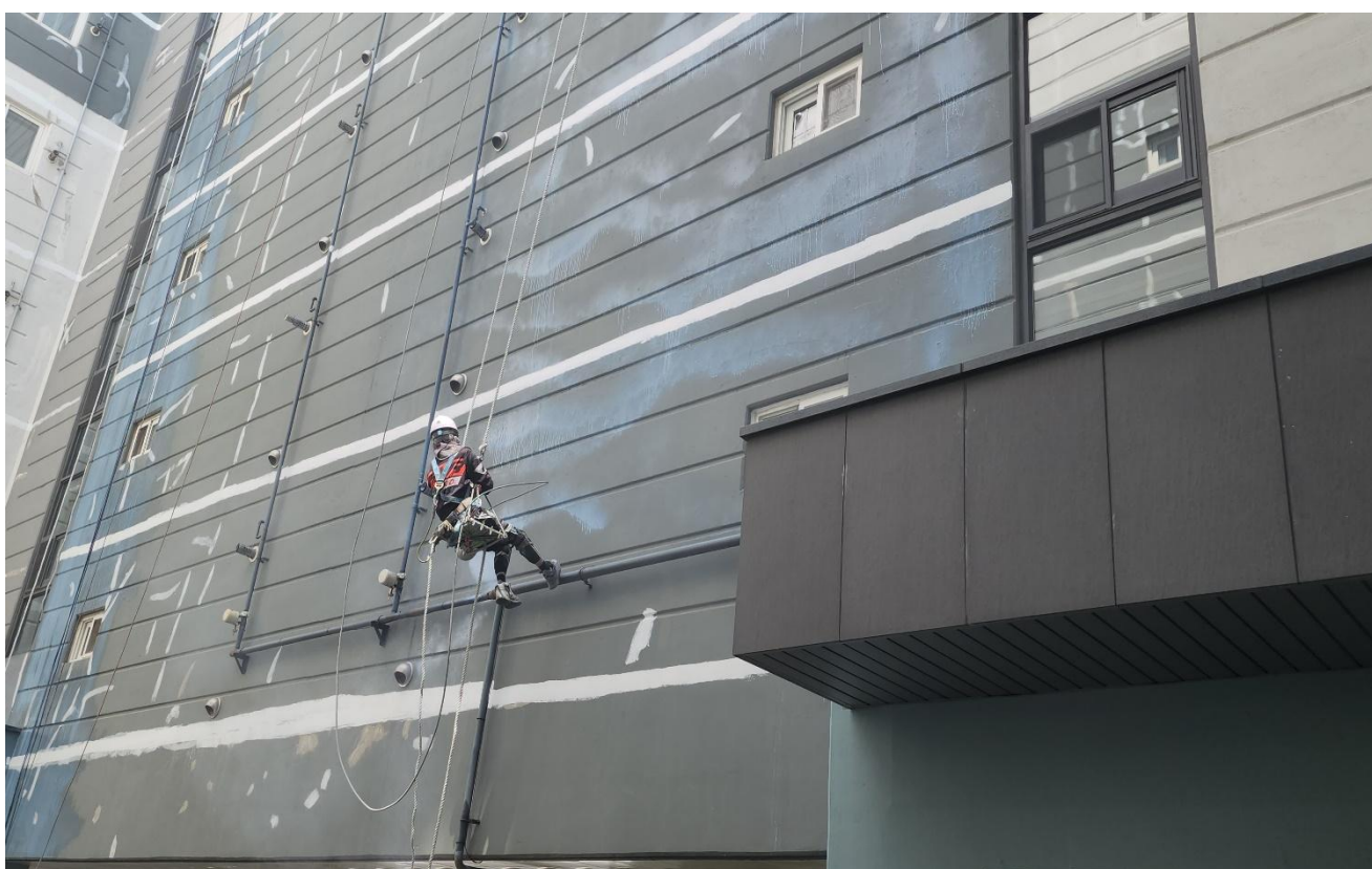
공사 중 (외부 : 바인다 도포)
