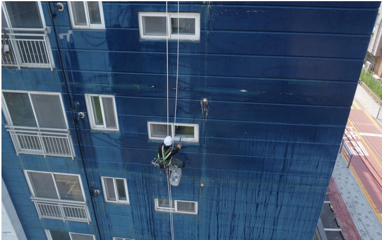
공사 중 (외부 : 고압세척)
