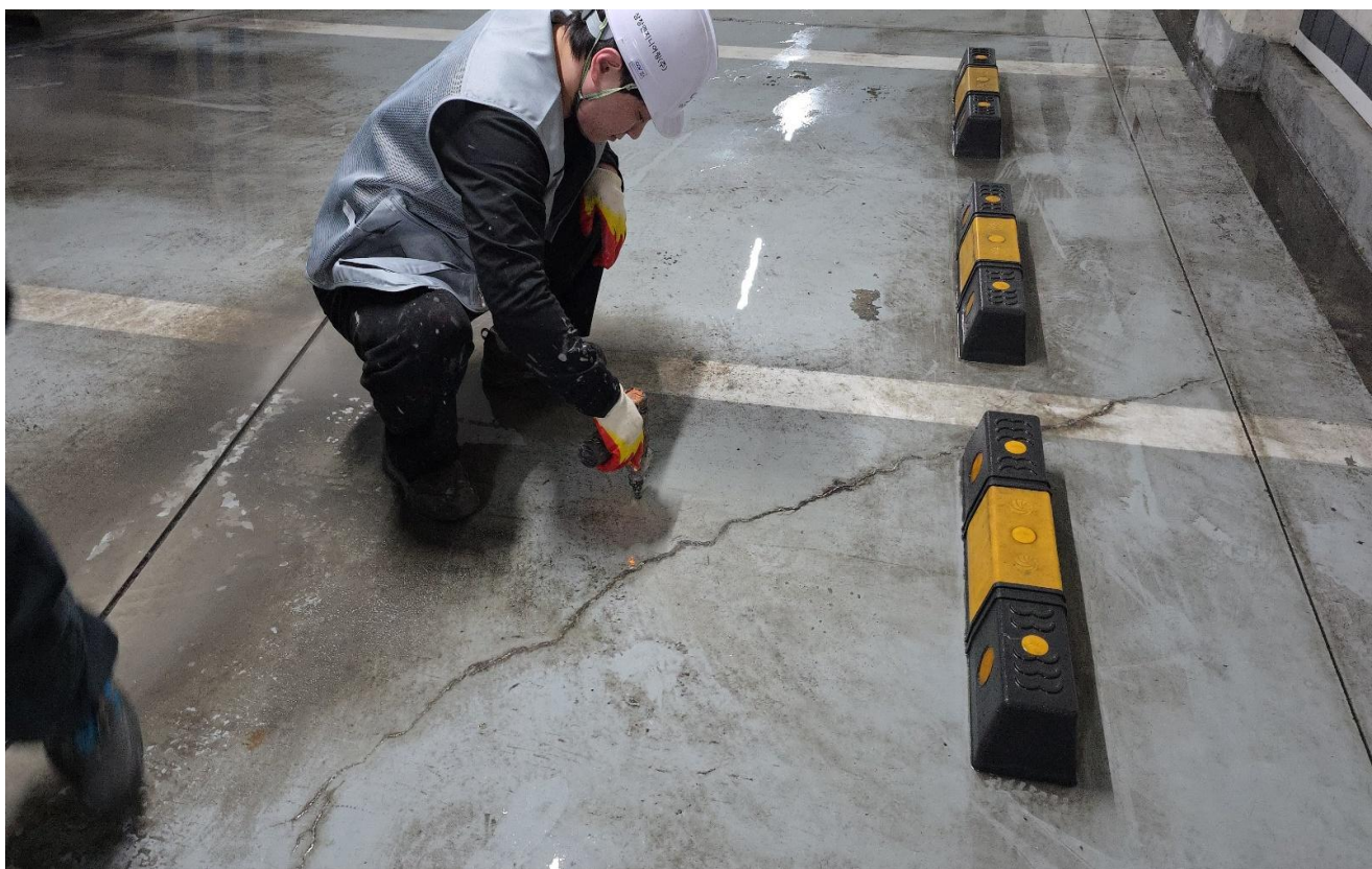
공사 중 (지하주차장 : 인젝션)
