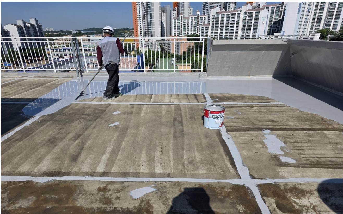
공사 중 (옥상 : 우레탄 중도 1차)
