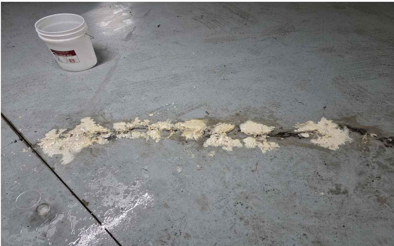
공사 중 (지하주차장 : 인젝션)
