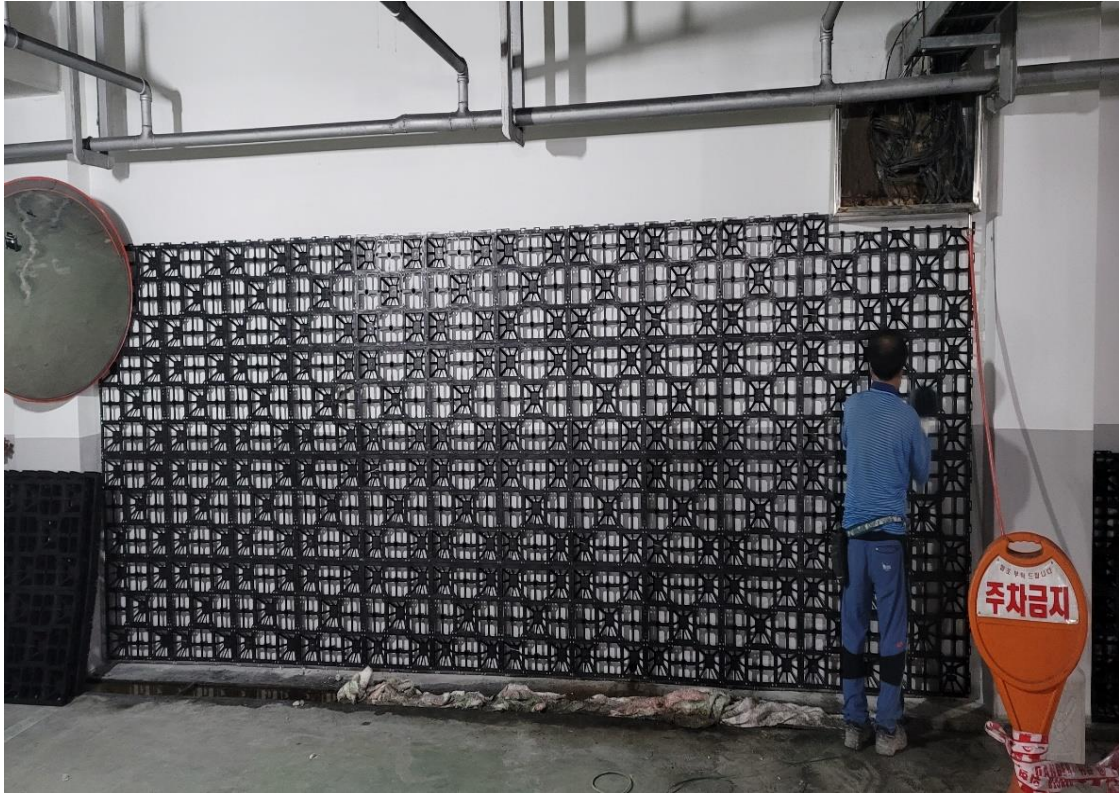
벽체 배수판 설치 작업중
