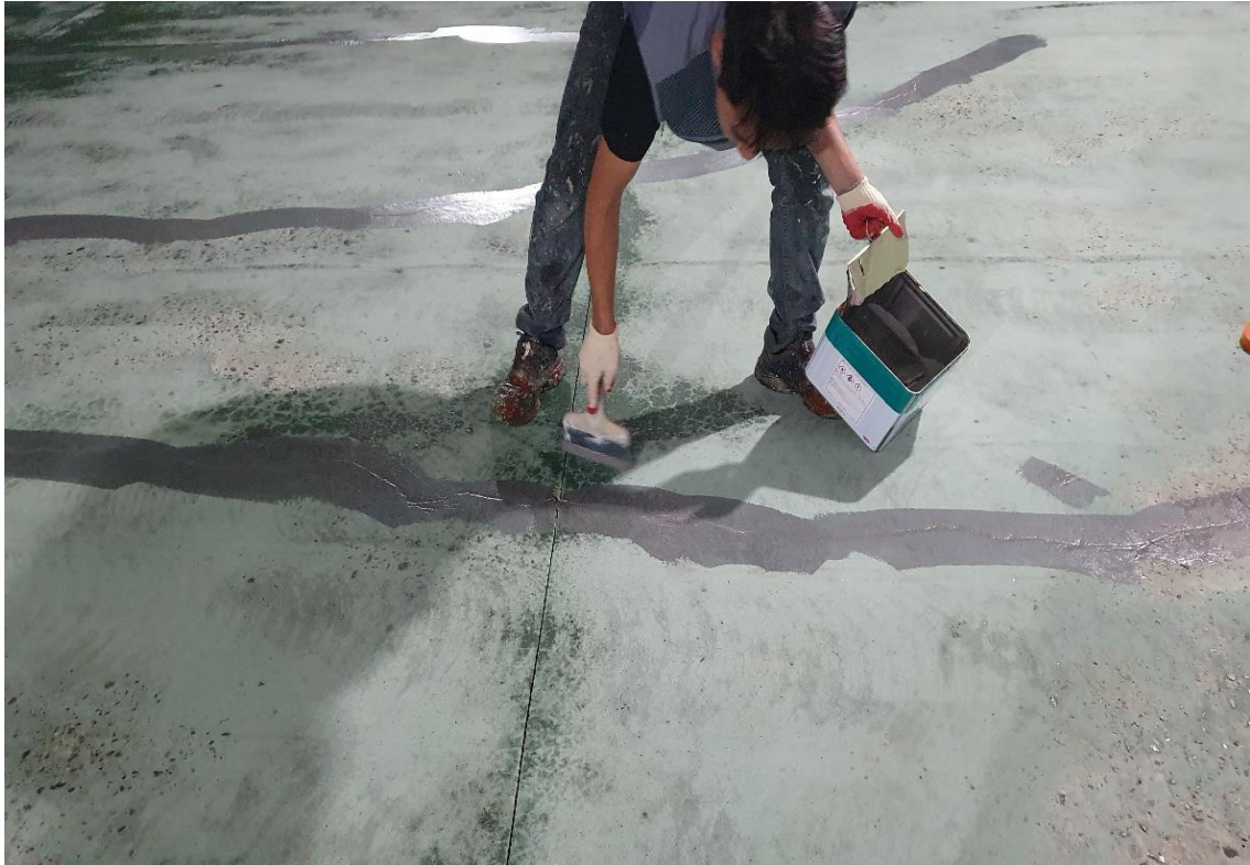
바닥 균열보수 작업중
