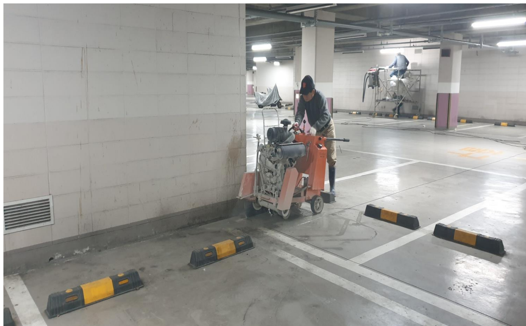
지하2층 트렌치 차수공법 시공
