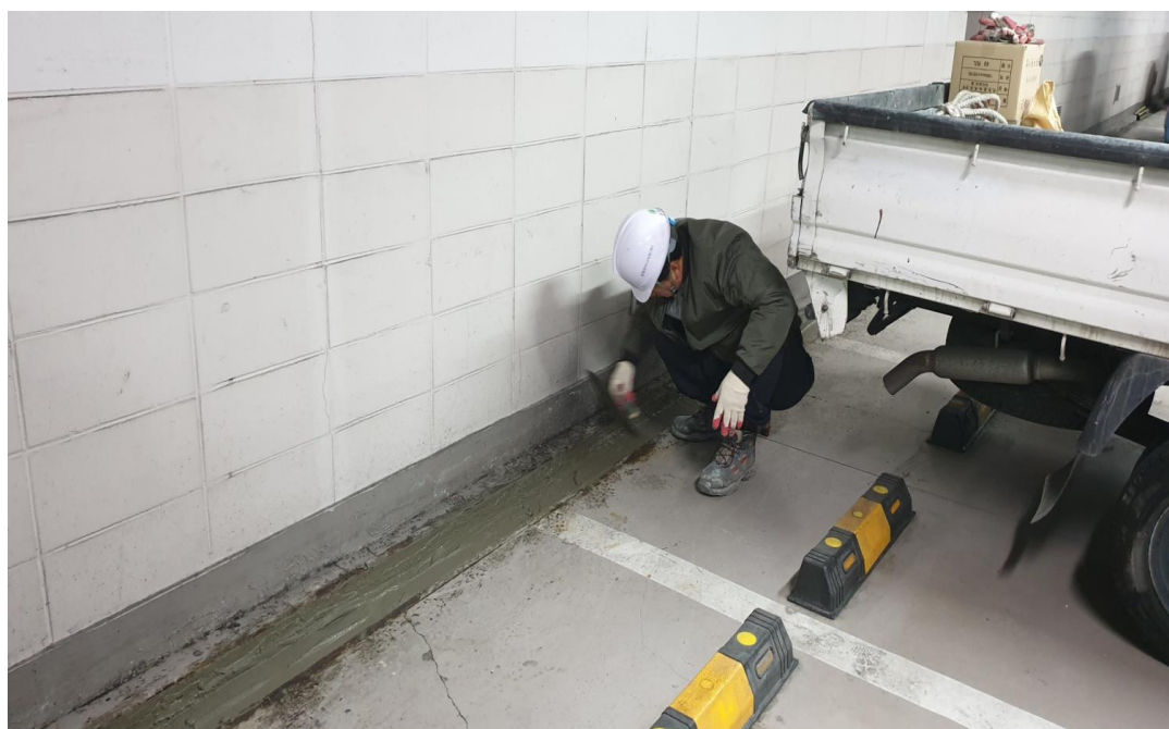
지하주차장 트렌치부위 액체방수 및 배관보수
