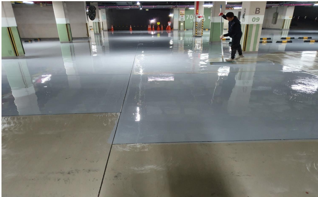
주차장 바닥 전체 무용제 도포
