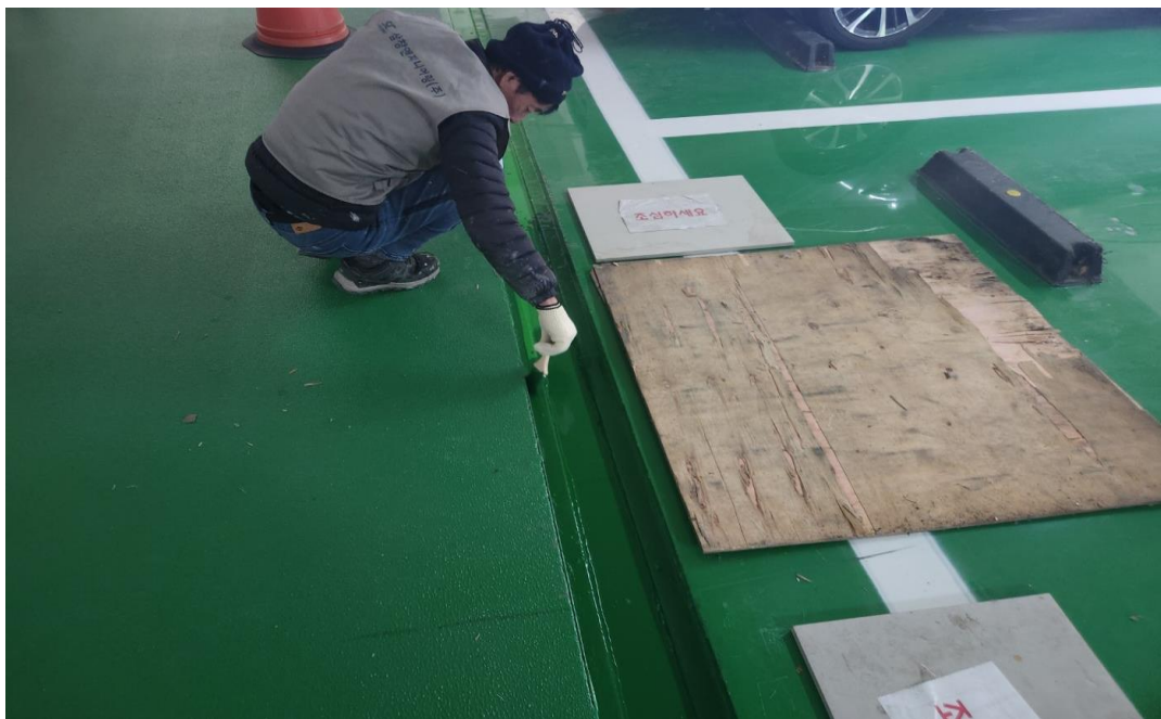
공사 중 (우레탄 시공)
