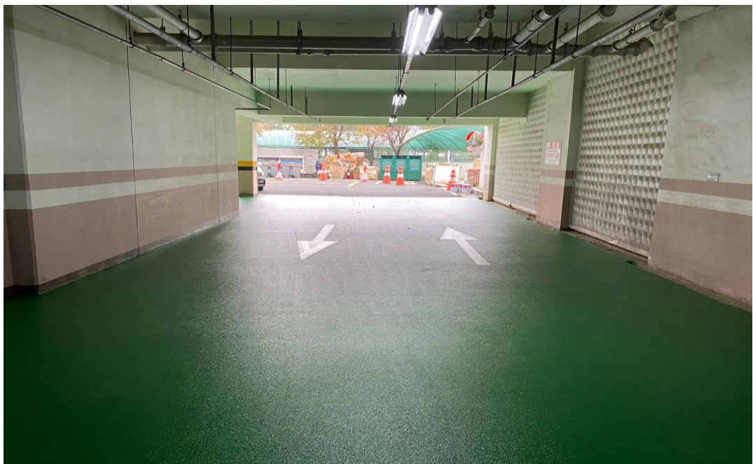
공사 후 (지하1층 공사완료)
