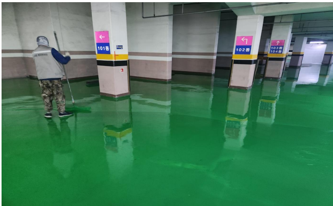
공사 중 (에폭시 중도 2차)
