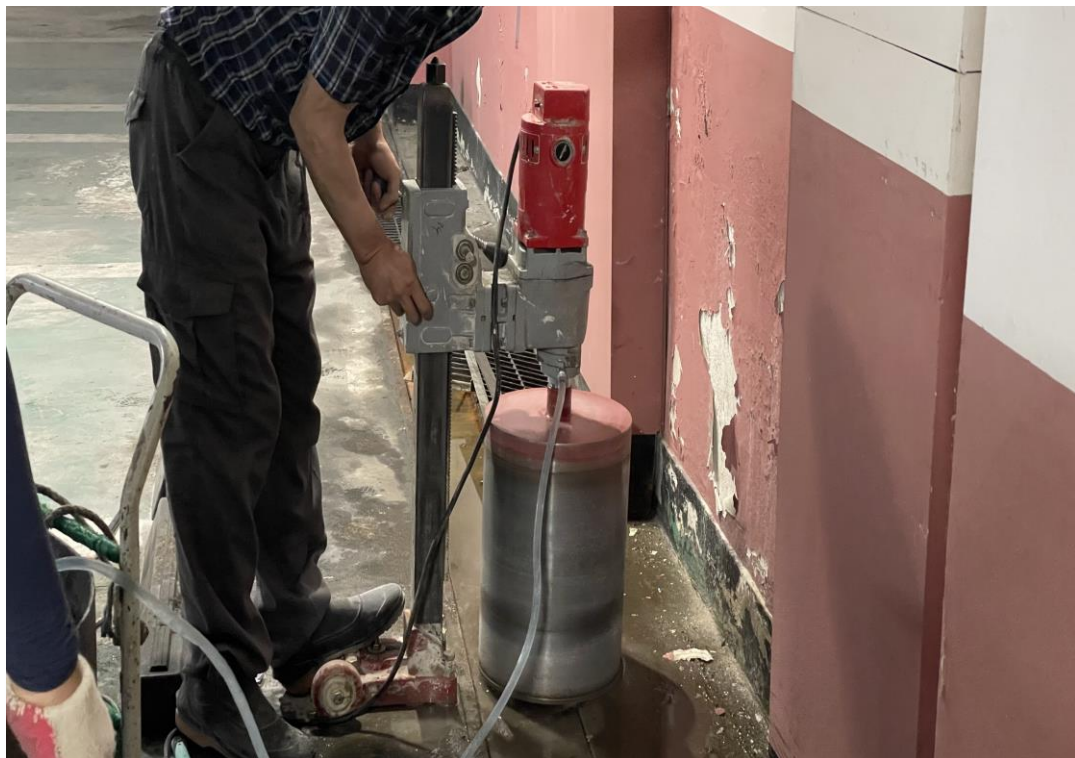
집수정 코아천공
