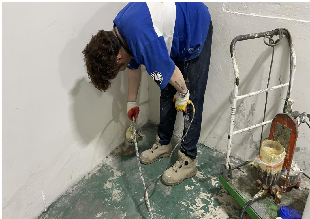
벽체 누수부위 고강도 발포우레탄 주입
