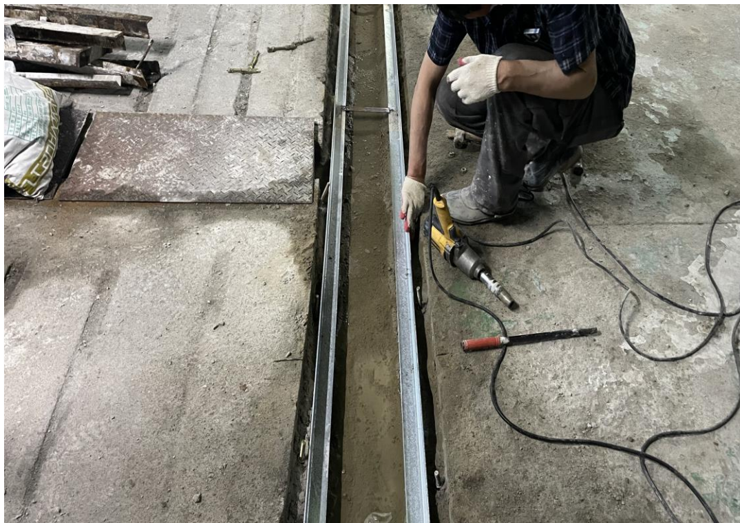
무소음 트랜치 양카 시공 및 앵글 설치
